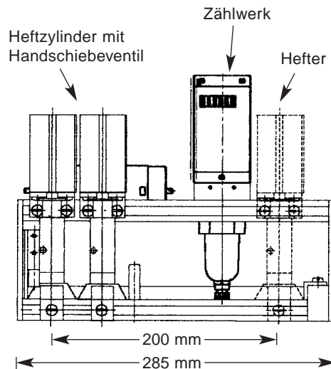
TH 210/3 pneumatisch
